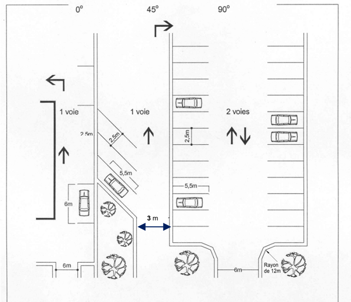
Croquis 8 : Dimension d'une case de stationnement
